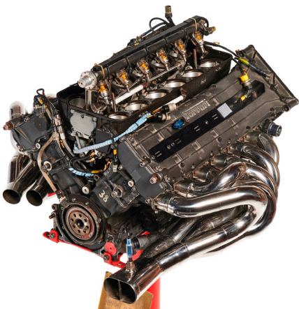
Exceptionnel moteur type Ferrari 3000 (044/1) pour Ferrari F412 T2, saison 1995 Adjugé 169 000 € / 203 628 $ frais inclus
