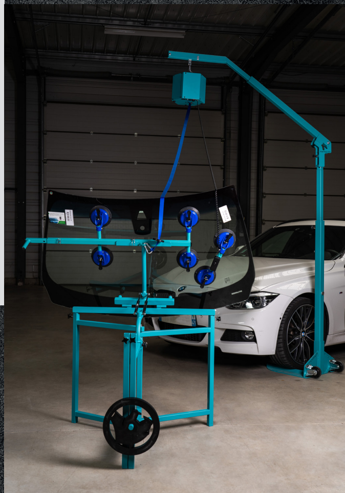
KIT FITGLASS ET SA TABLE MODULABLE PPP-WST210N2
