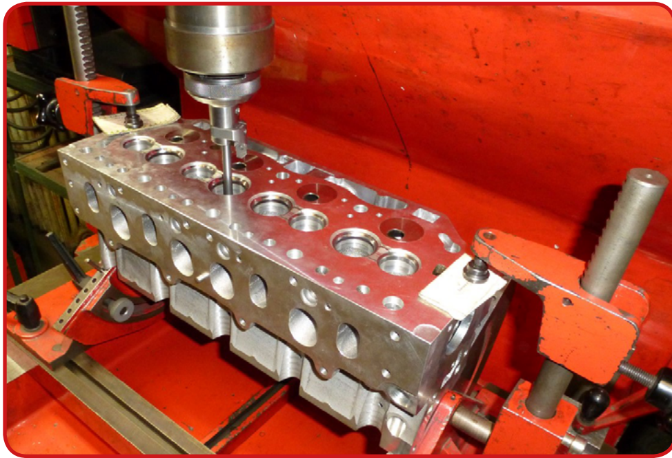
Intervention sur une culasse
